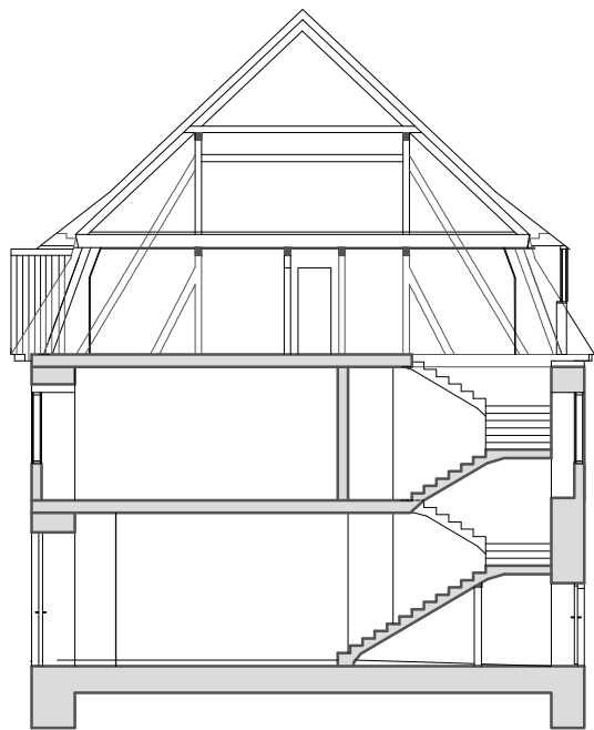
QUERSCHNITT
