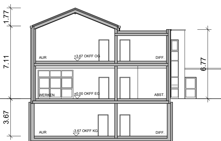
QUERSCHNITT
